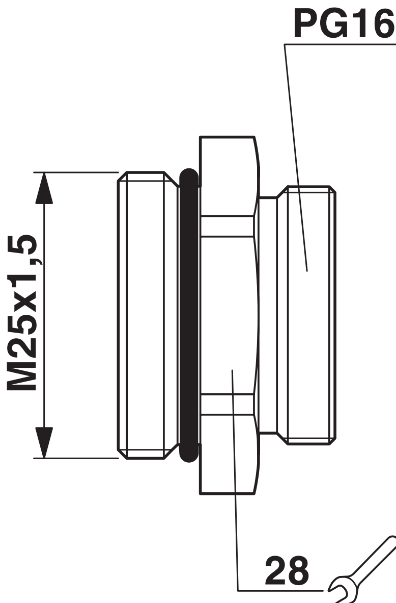
Rysunek wymiarowy
