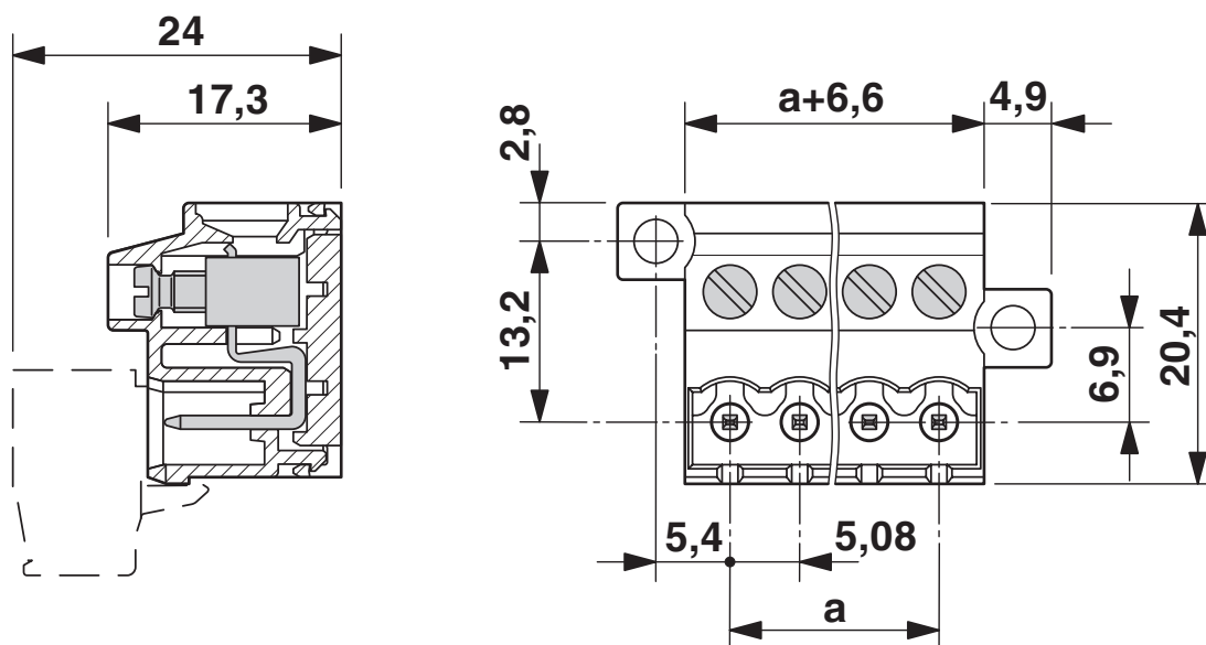
Rysunek wymiarowy
