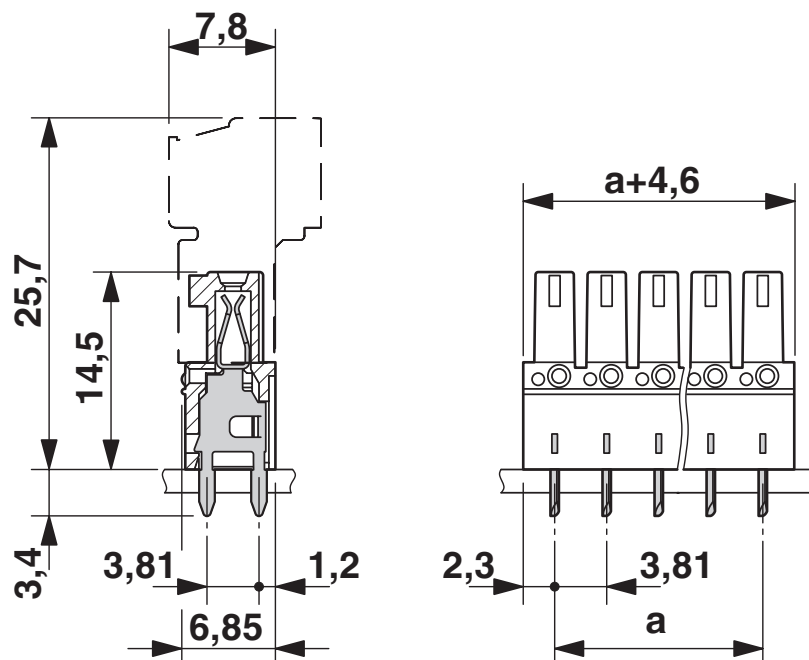
Rysunek wymiarowy
