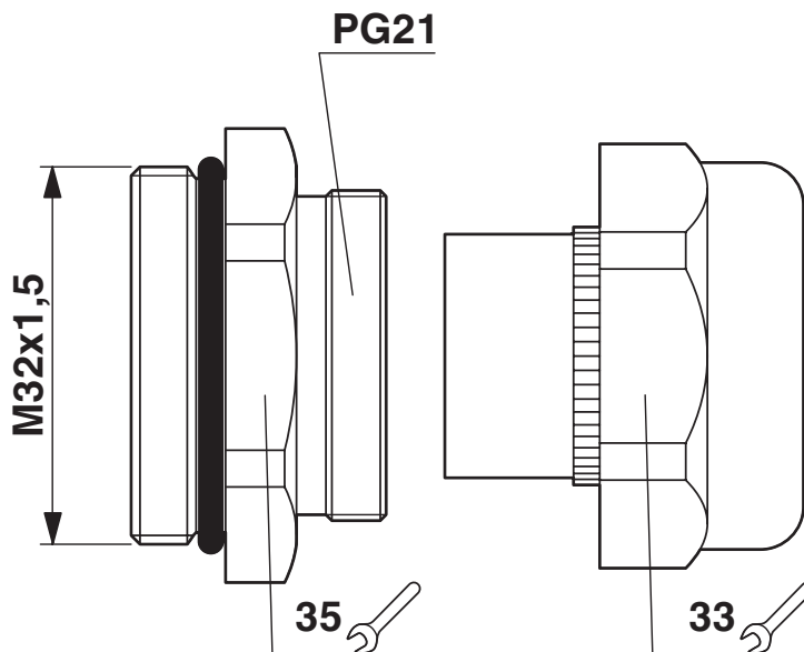
Rysunek wymiarowy
