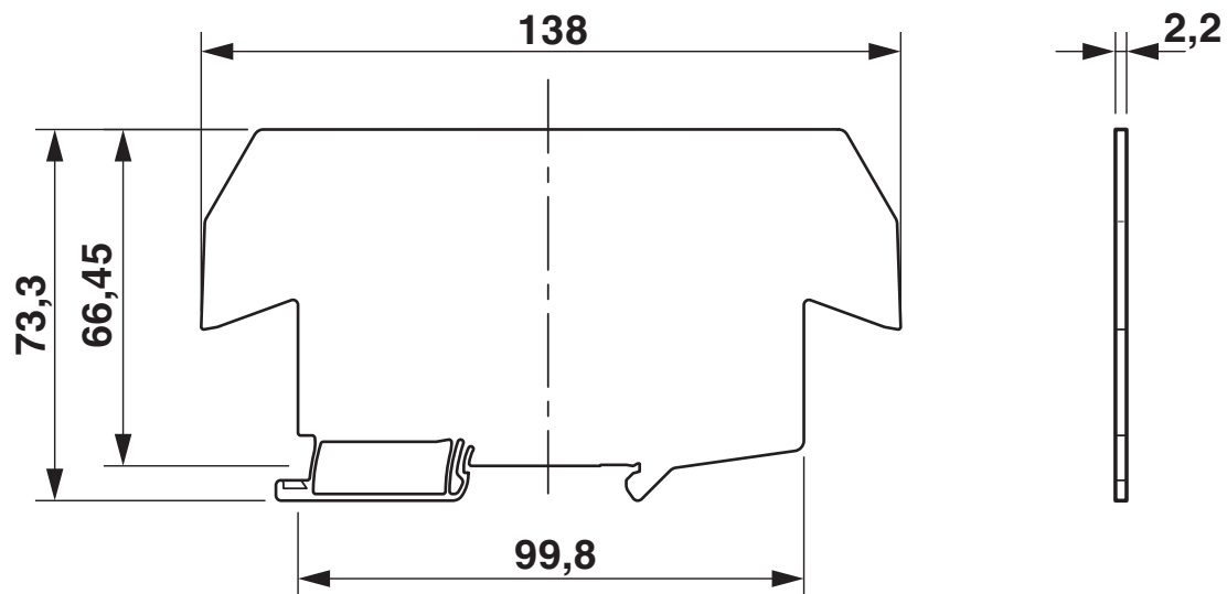
Rysunek wymiarowy
