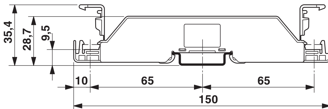
Rysunek wymiarowy
