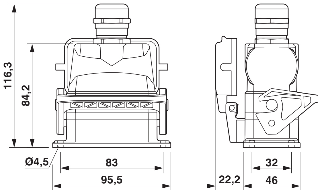
Rysunek wymiarowy
