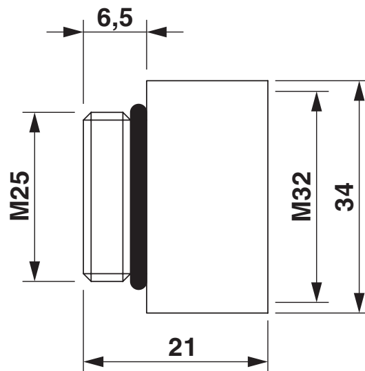
Rysunek wymiarowy
