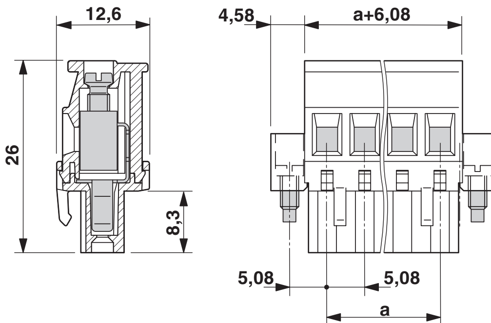
Rysunek wymiarowy
