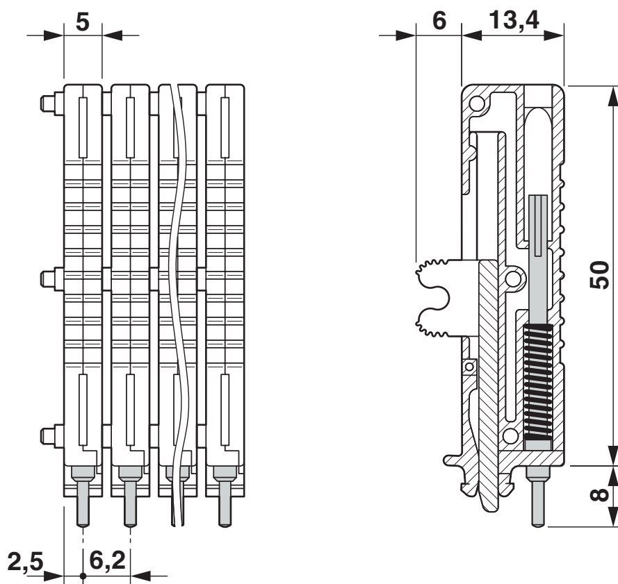
Rysunek wymiarowy
