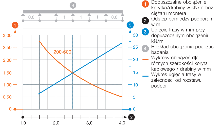
Wykres obciążenia drabiny typ SLG 45 NS
