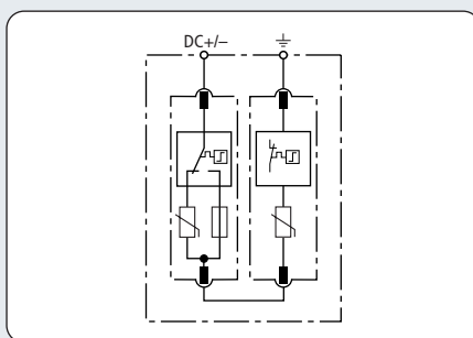
Schemat połączeń DG S PV SCI ...
