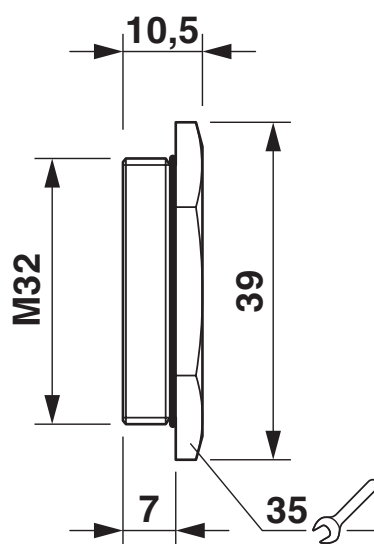
Rysunek wymiarowy
