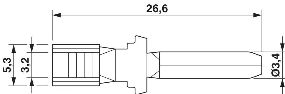
Rysunek wymiarowy
