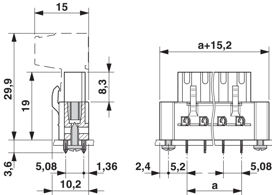
Rysunek wymiarowy
