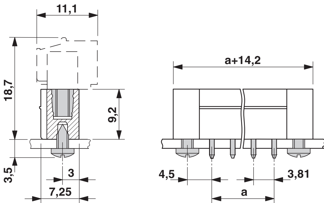
Rysunek wymiarowy
