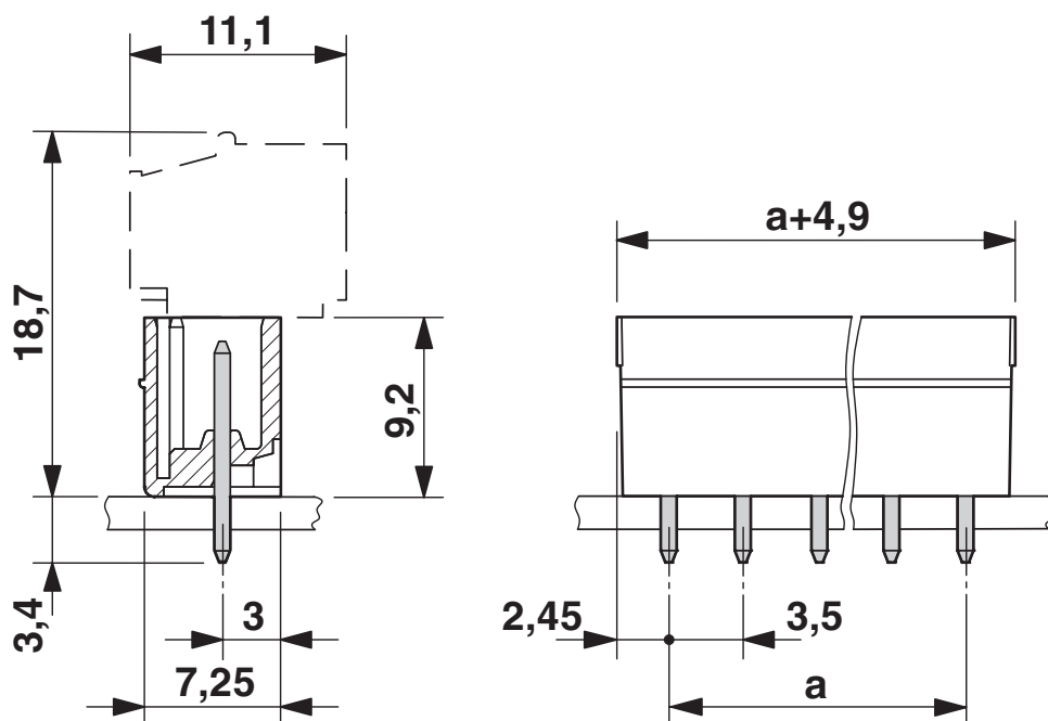
Rysunek wymiarowy
