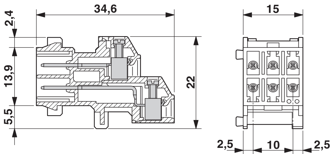
Rysunek wymiarowy
