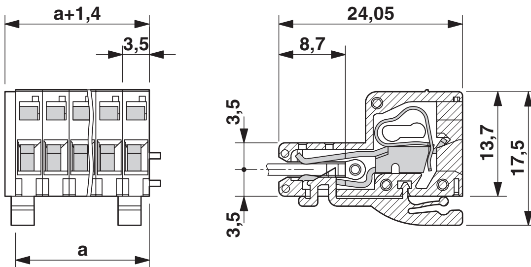
Rysunek wymiarowy
