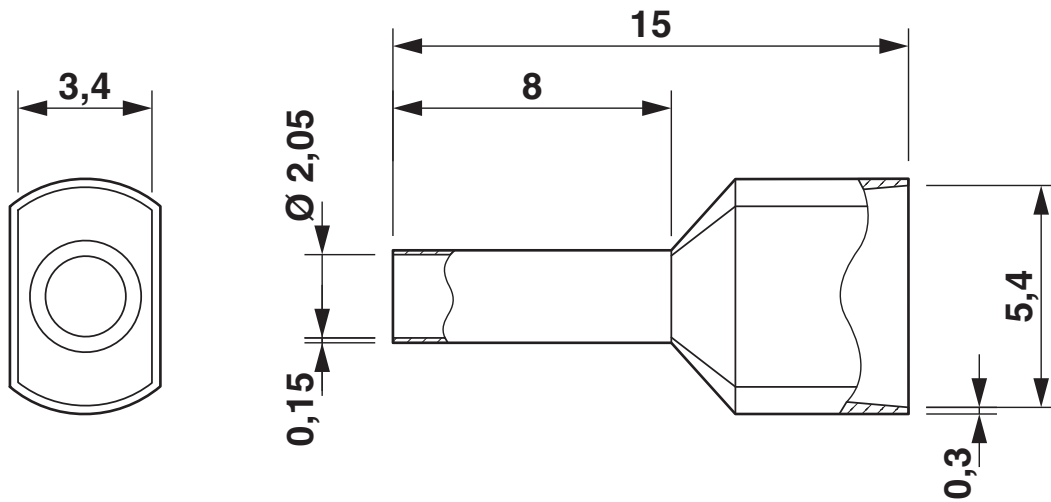
Rysunek wymiarowy
