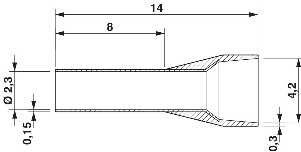
Rysunek wymiarowy
