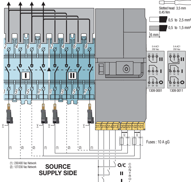
LOAD SIDE
