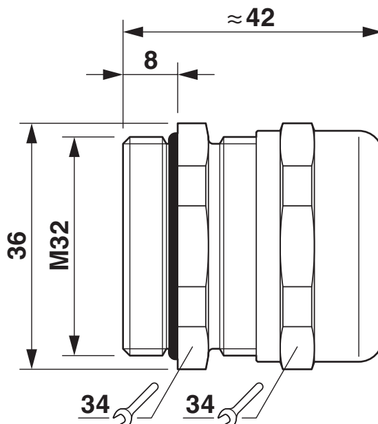
Rysunek wymiarowy
