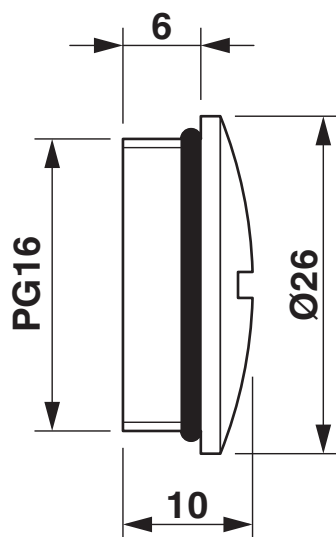
Rysunek wymiarowy
