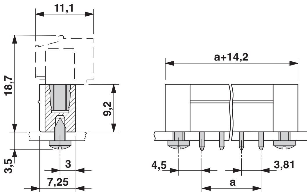
Rysunek wymiarowy
