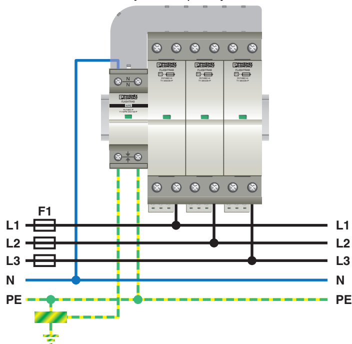
rysunek aplikacji
