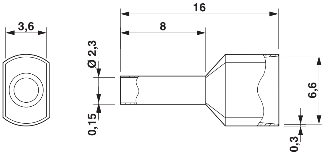
Rysunek wymiarowy
