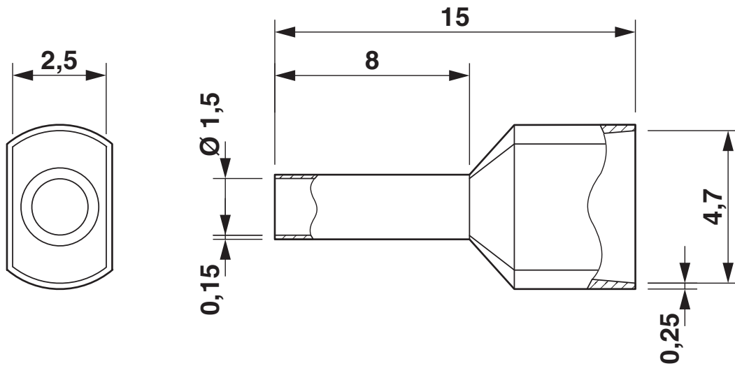
Rysunek wymiarowy
