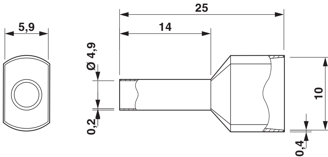
Rysunek wymiarowy
