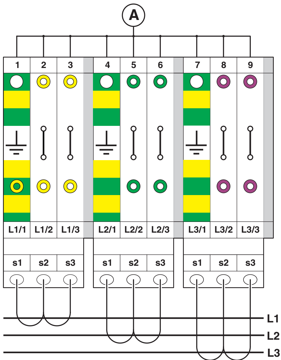
rysunek złączy
