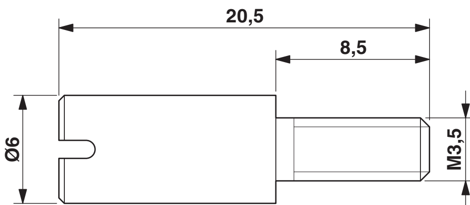
Rysunek wymiarowy
