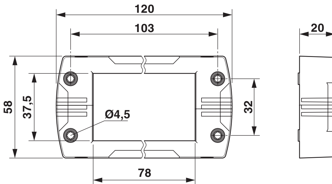
Rysunek wymiarowy
