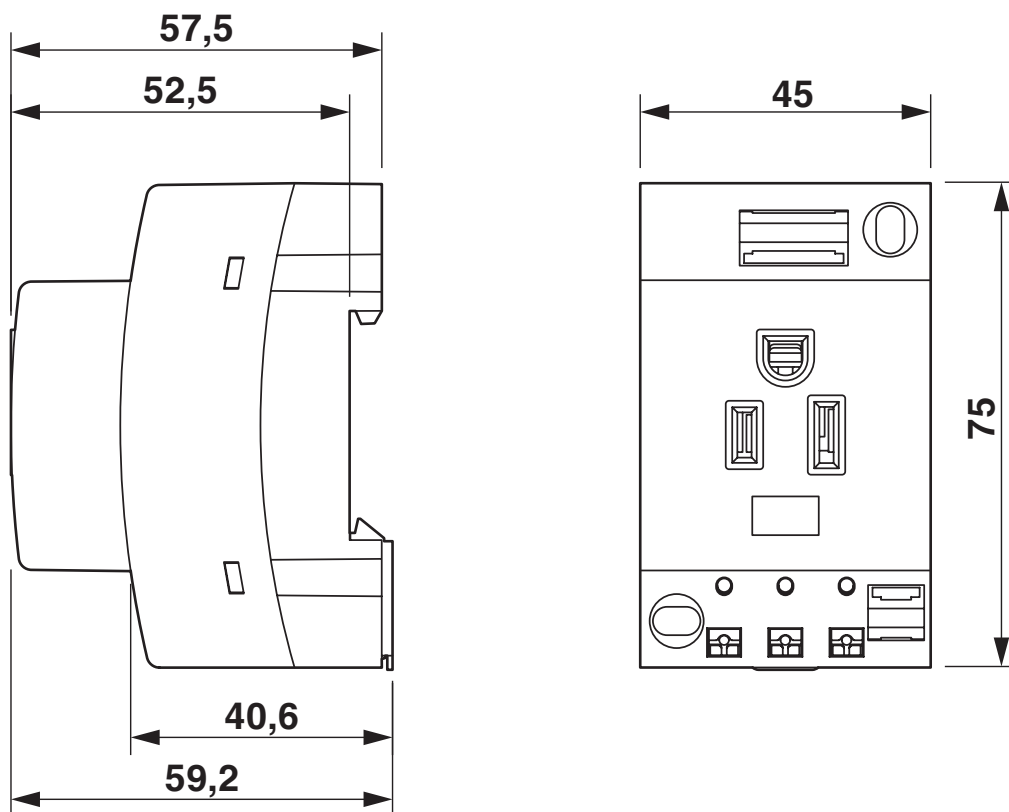
Rysunek wymiarowy
