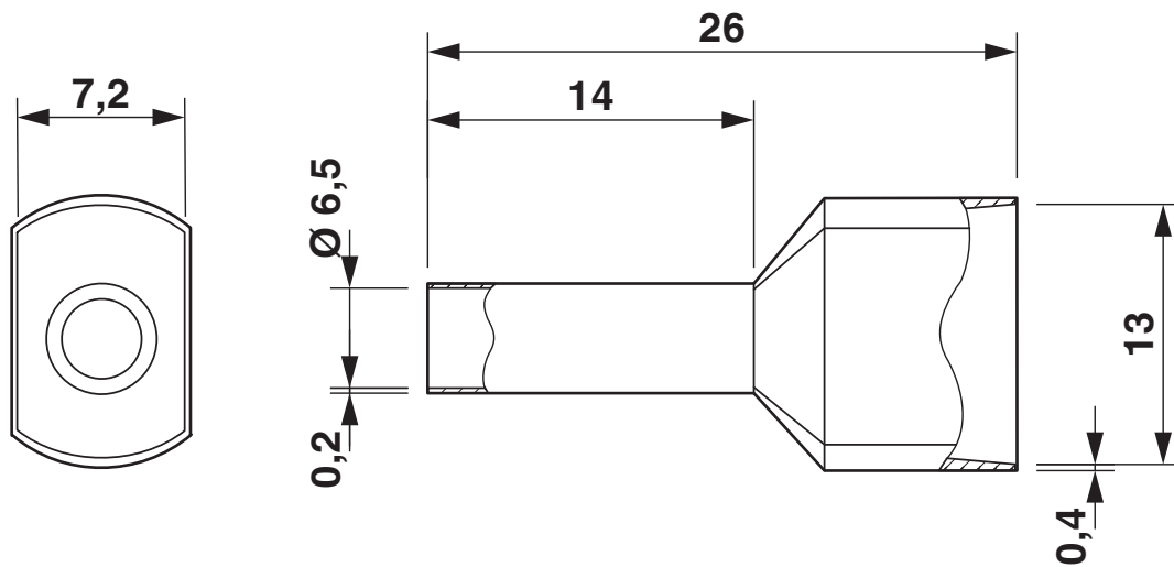
Rysunek wymiarowy
