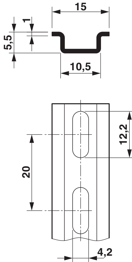
Rysunek wymiarowy
