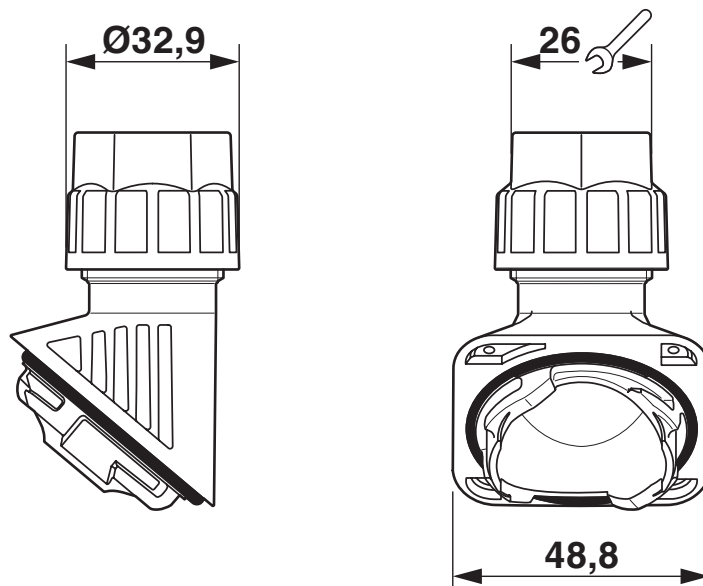
Rysunek wymiarowy
