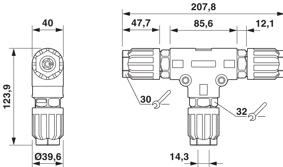
Rysunek wymiarowy
