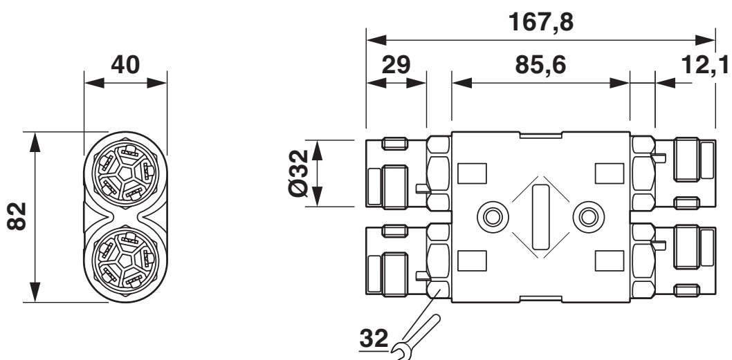
Rysunek wymiarowy
