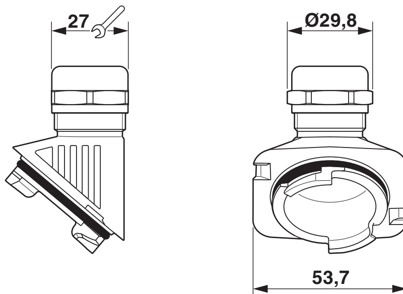
Rysunek wymiarowy
