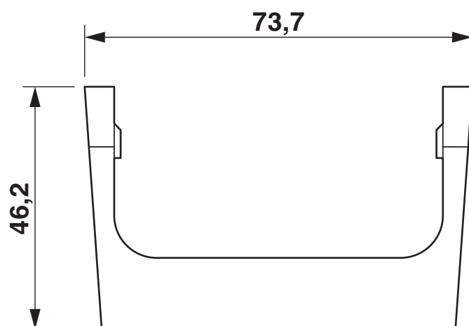
Rysunek wymiarowy
