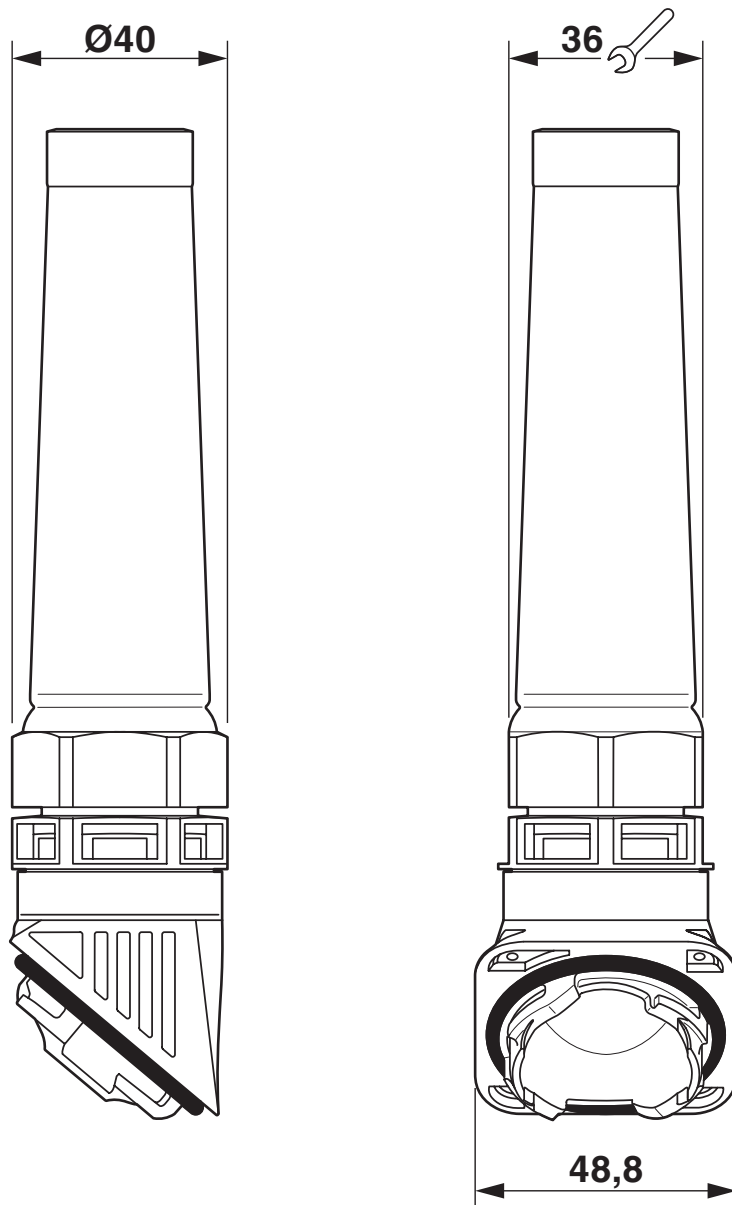
Rysunek wymiarowy
