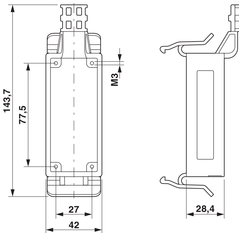
Rysunek wymiarowy
