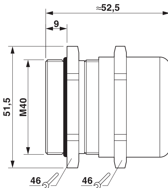
Rysunek wymiarowy
