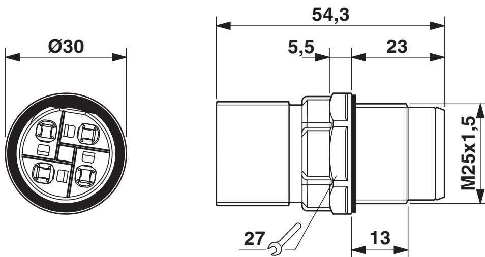
Rysunek wymiarowy
