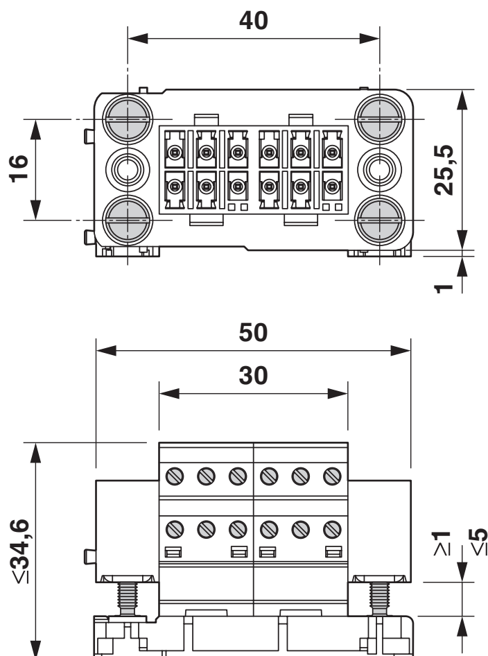
Rysunek wymiarowy
