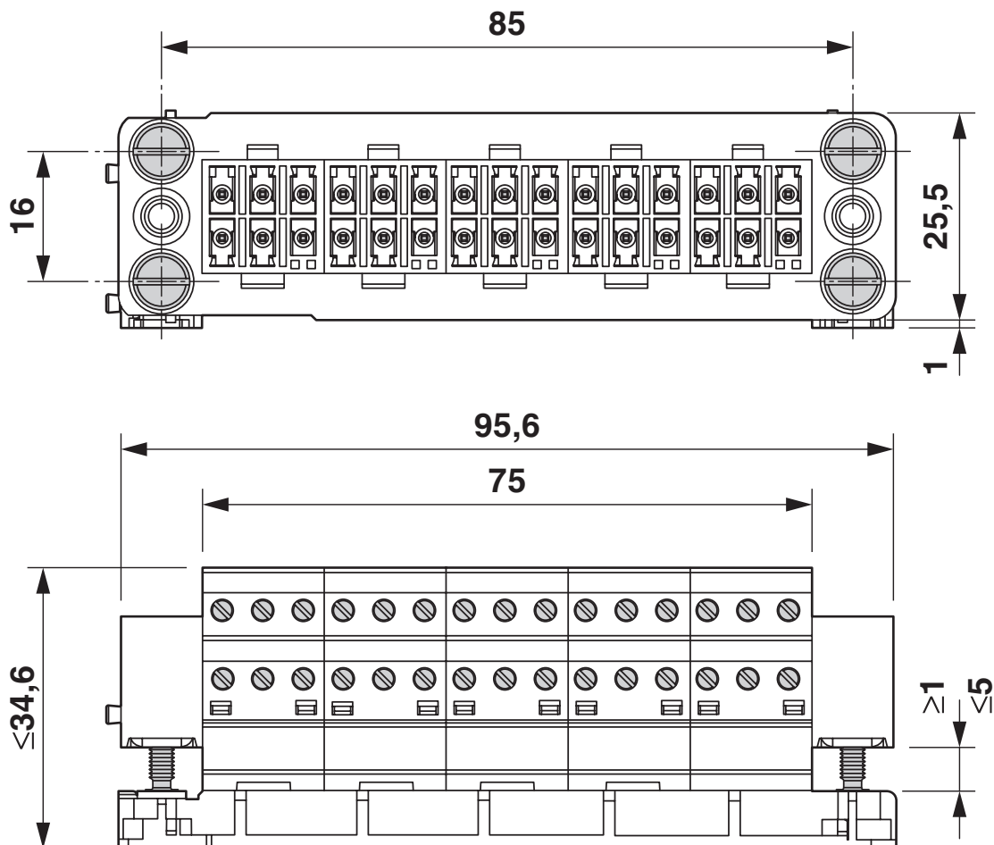
Rysunek wymiarowy
