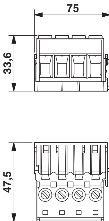
Rysunek wymiarowy
