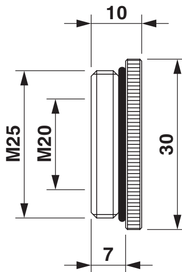
Rysunek wymiarowy
