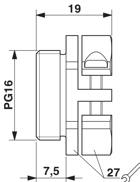
Rysunek wymiarowy
