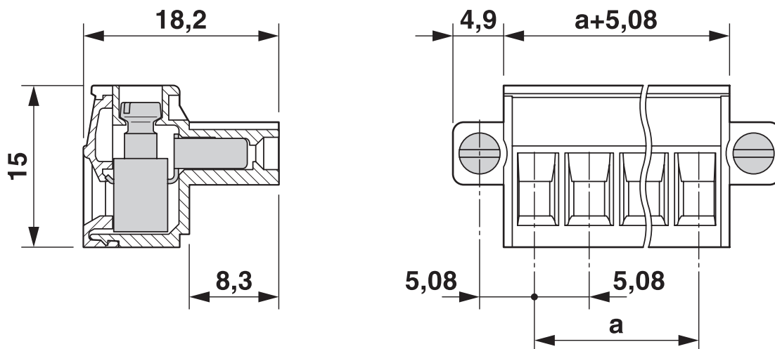
Rysunek wymiarowy
